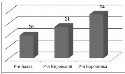
Гистограмма 1. Уровень загрязнения воздуха окисью углерода K_{co} , mg/m^3
