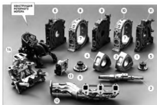
Рис. 2. Конструкция роторно-поршневого двигателя внутреннего сгорания 1 – внутренняя шестерня ротора; 2 – передний ротор; 3 – эксцентриковый вал; 4 – задний ротор; 5 – стационарная (неподвижная) шестерня; 6 – задний корпус (боковой); 7– отверстия свечей зажигания; 8 – корпус заднего ротора(статор); 9 – промежуточный корпус(боковой); 10 – корпус переднего
