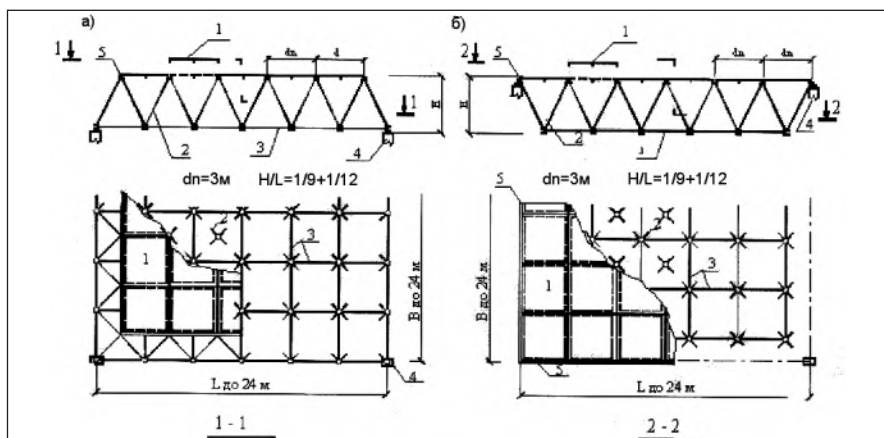
Рис. 2. Схемами оперения структурных плит
