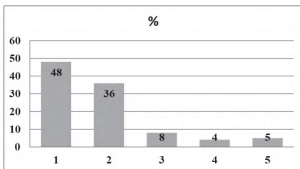
Рис. 4. Гистограмма распределения причин отказов гидросистем СТ и СДМ: 1 – внешняя негерметичность; 2 – внутренняя негерметичность; 3 – нарушение функционирования агрегата; 4 – разрушение элементов агрегата; 5 – прочие отказы
